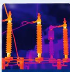
DAO CÁCH LY, CHỐNG SÉT
